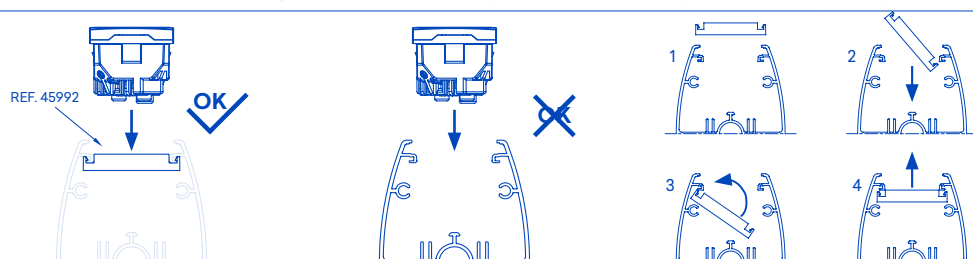
REF. 45992 - ESQUEMA DE MONTAGEM | ESQUEMA DE MONTAJE | MOUNTING DIAGRAM | SCHÉMA DE MONTAGE | EINBAUPLAN
